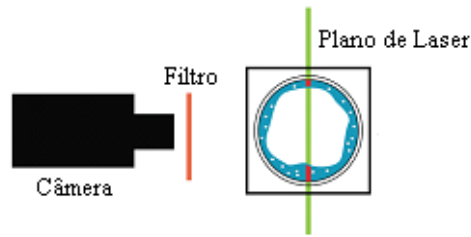
Figura 1: Visão esquemática do arranjo óptico montado
