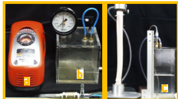
Figura 2: Aparato desenvolvido para bombeamento suave, registro e controle da pressão interna, pressurizador(a), recipiente primário (b), recipiente com água sob pressão(c).
