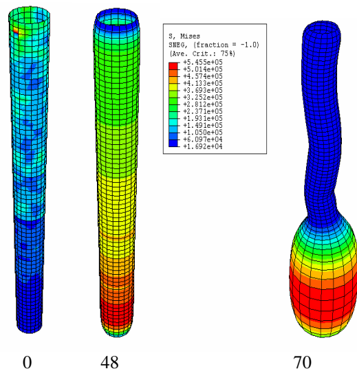
Figura 4: Sequência da pressurização do tubo de silicone sem tração, pressões em (mmHg).
