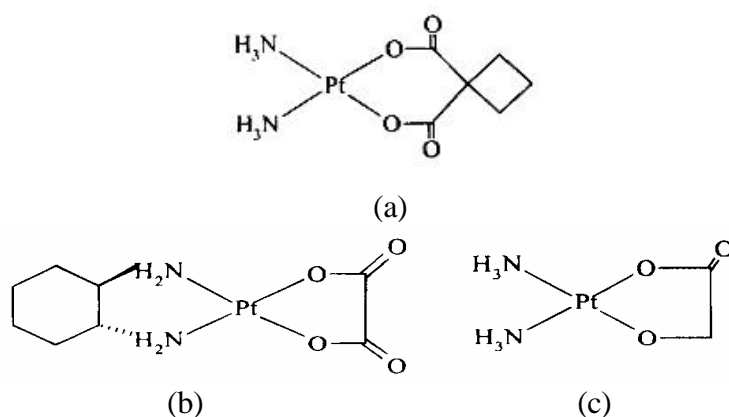
Figura 2 - Fórmula estrutural dos análogos de platina de 2 a geração: carboplatina (a), oxaliplatina
