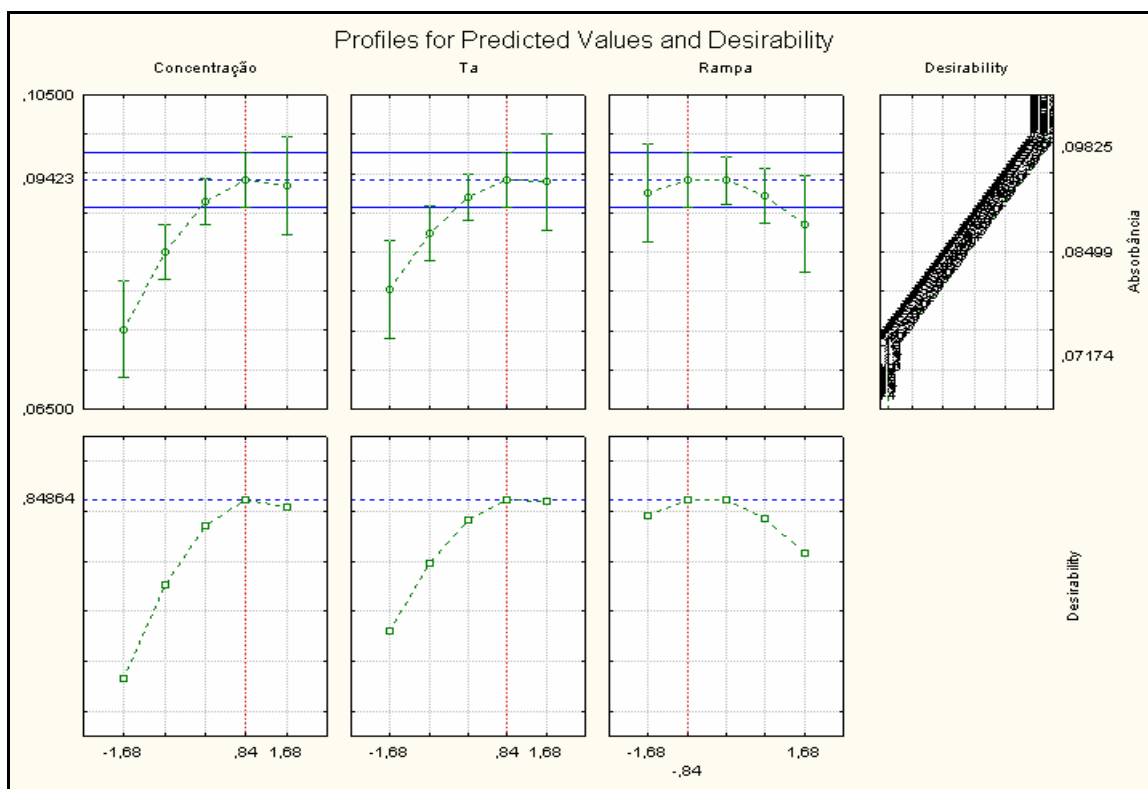
Figura 12: Perfil dos valores previstos/otimizados e da desejabilidade para o planejamento composto central.
